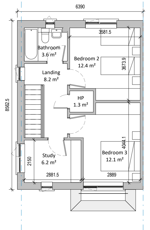
④ H08L Level 02 1 : 100
